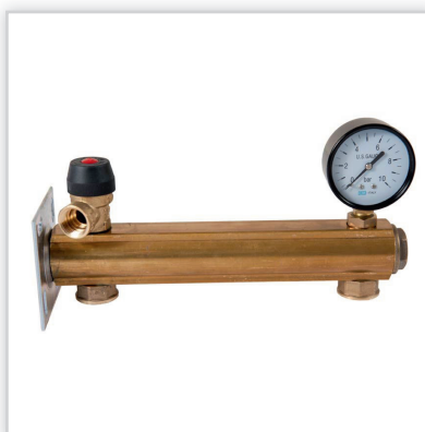
Grupa bezpieczeństwa do C.W.U. (ciepła woda użytkowa) z zaworem bezpieczeństwa 6 bar.
