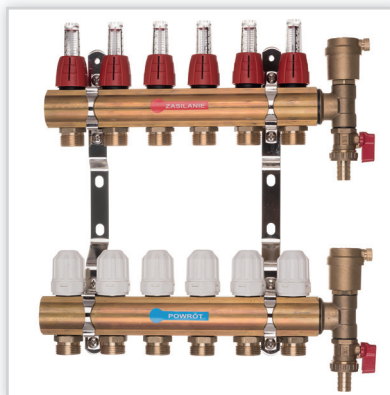
Rozdzielacz CD 473 Rozdzielacz mosiężny do ogrzewania podłogowego 1'' z przepływomierzami i wkładkami zaworowymi M30 x 1,5 oraz sekcją odpowietrznikowo-spustową.
