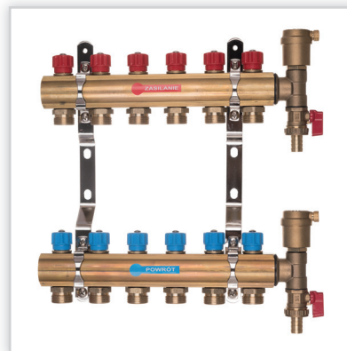
Rozdzielacz CDR Rozdzielacz mosiężny do ogrzewania podłogowego 1'' z manualnymi zaworami odcinającymi oraz sekcją odpowietrznikowo-spustową.
