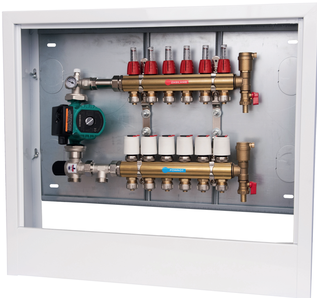
Zestaw do ogrzewania podłogowego z grupą mieszącą z rozdzielaczem ze wskaźnikami przepływów i siłownikami termicznymi
